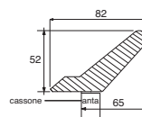
sezione cornice frame cross-section
